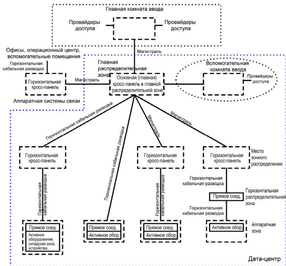
Рис. 2. Топология дата-центра
