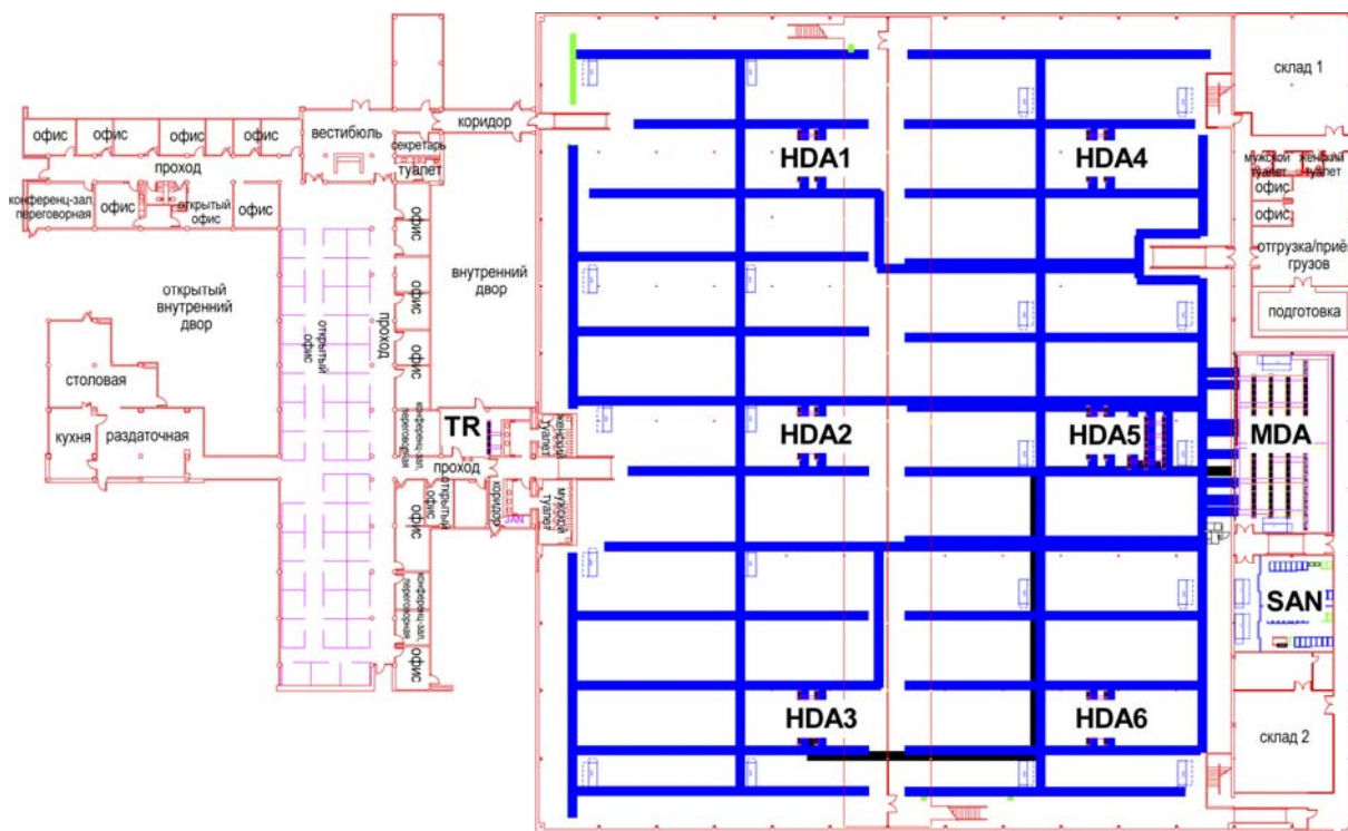
Рис. 22. Пример Интернет дата-центра
